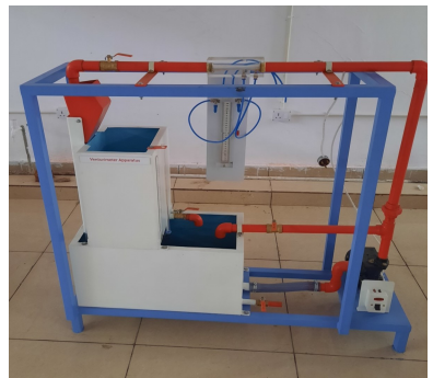
Venturimeter Apparatus
